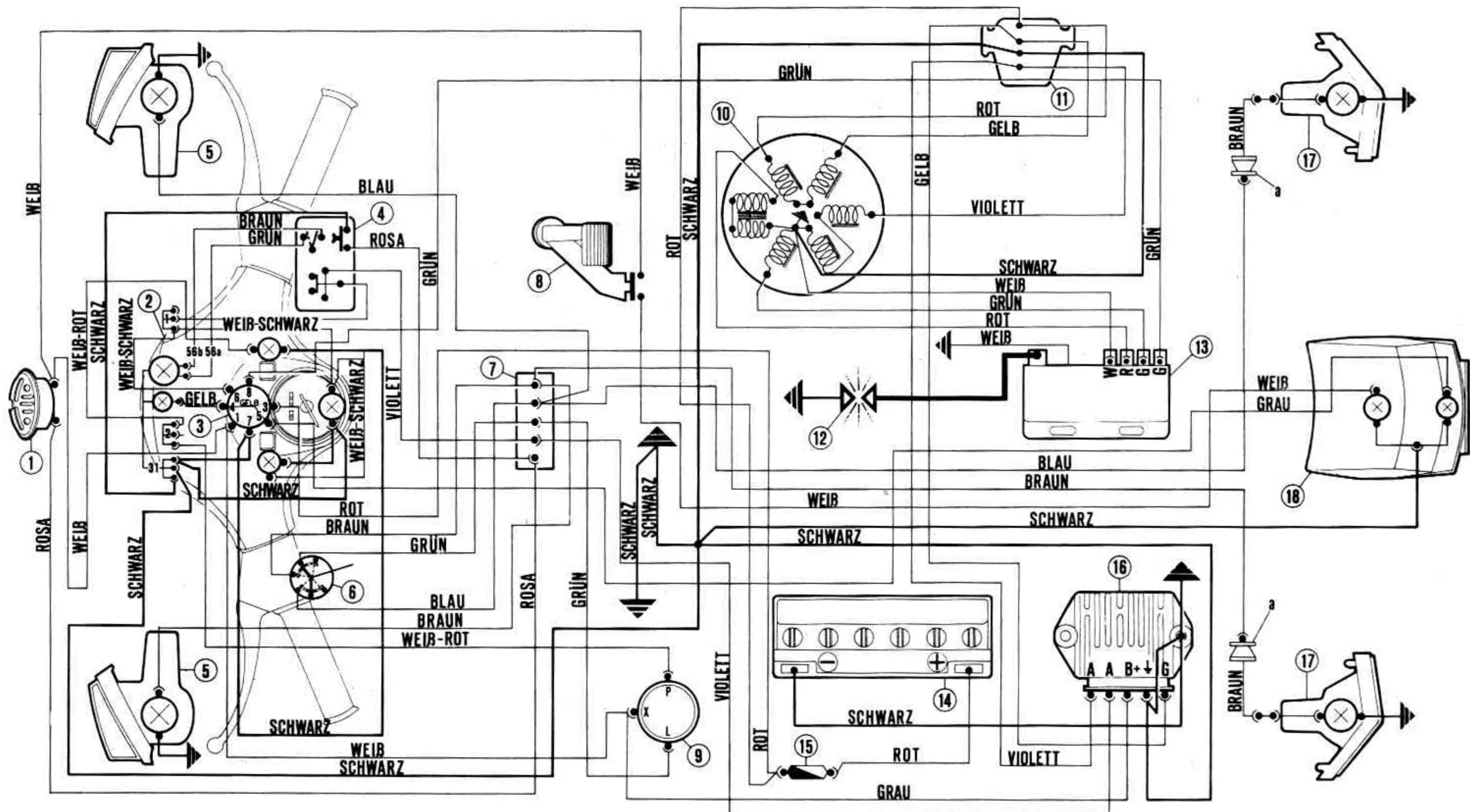
Schaltplan P 200 E (S. Abb., Seite 11).
