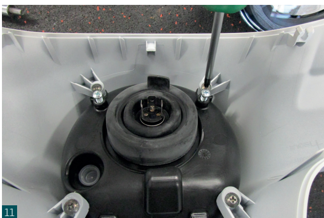
11 Scheinwerfer montieren. Mount headlight.
