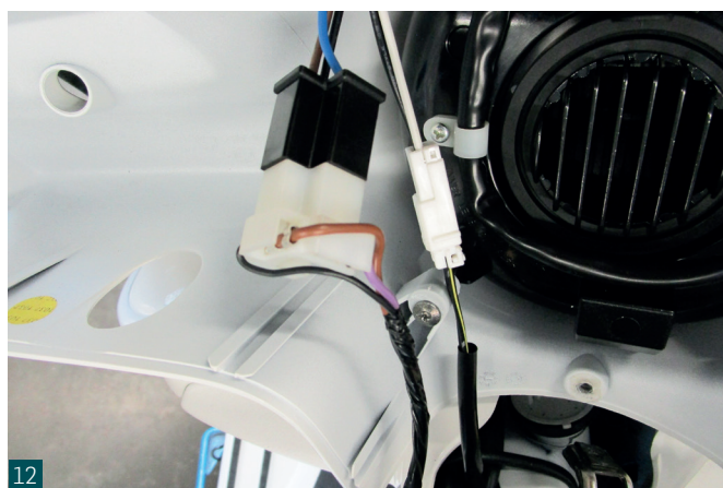
12 LED-Scheinwerfer einstecken. Anschließend erfolgt der Zusammenbau in umgekehrter Reihenfolge. Connect LED headlight. Reassembly in reverse order.
